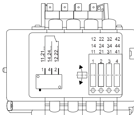
Abb. 15. 4-stufiger Getriebeendschalter
