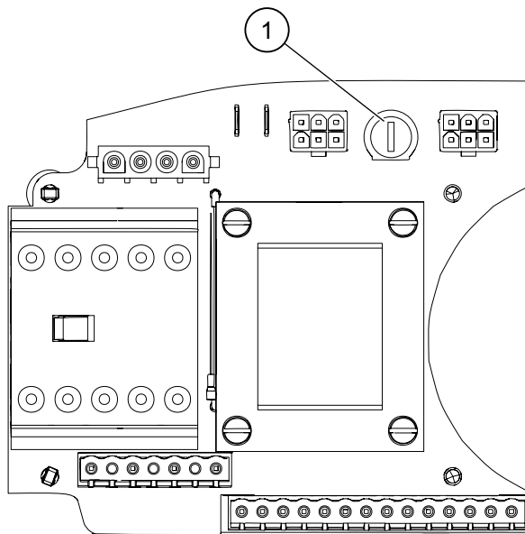
Abb. 18. Netzteileplatine mit Steuerspannungs-Sicherung
