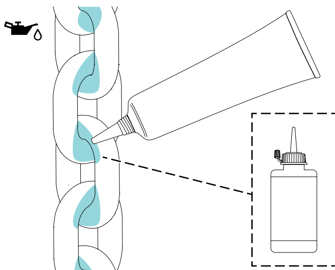
Abb. 20. Korrektes Positionieren des Schmierrohrs oder der Ölflasche
