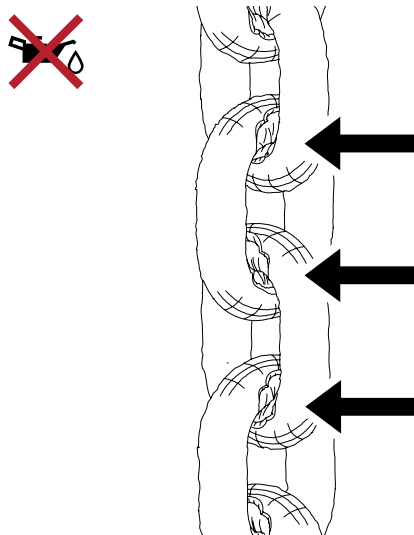
Abb. 22. Vollständig trockene und beschädigte Kette
