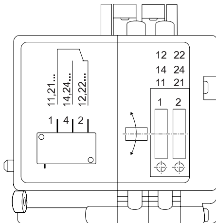
Abb. 9. 2-stufiger Getriebeendschalter
