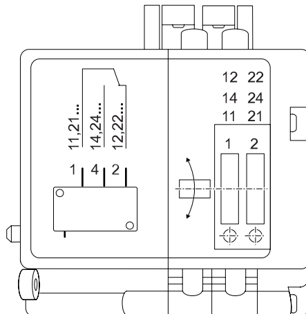
Abb. 14. 2-stufiger Getriebeendschalter
