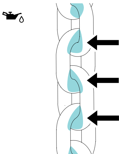
Abb. 19. Korrekte Schmierstellen an der Kette
